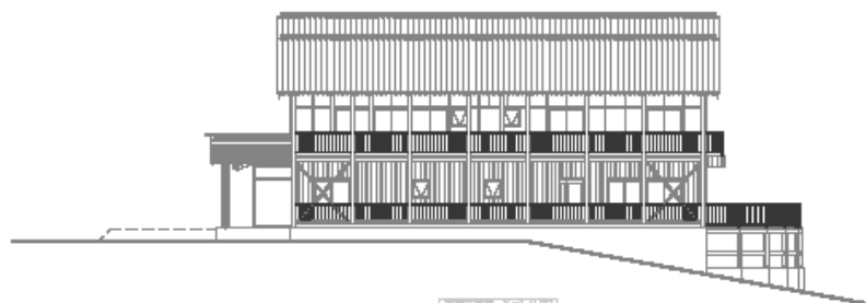
1.14. 立面図
