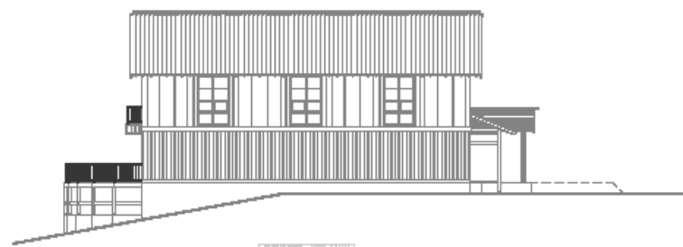
1.14. 立面図
